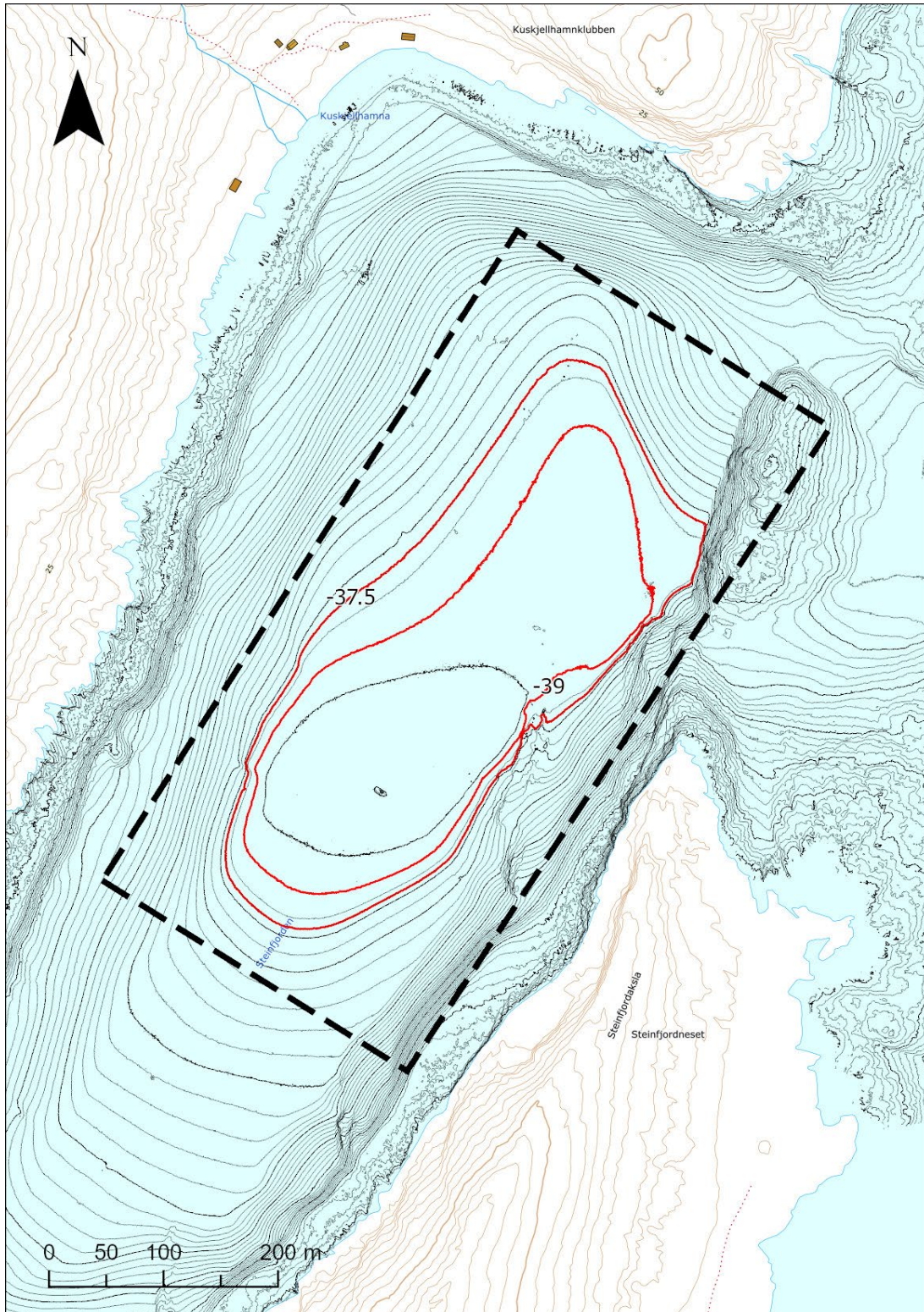
Plangrense, med dybdekoter. Kote for topp og bunn deponi er framhevet med rødt. (Multiconsult Norge)
