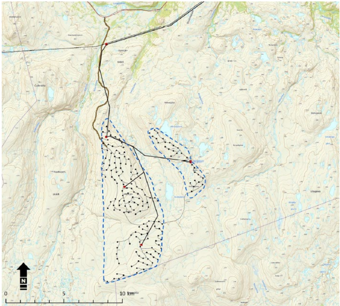
Govus 4-1: Davvi bieggafápmorusttega gaskaboddosaš huksenplána.
