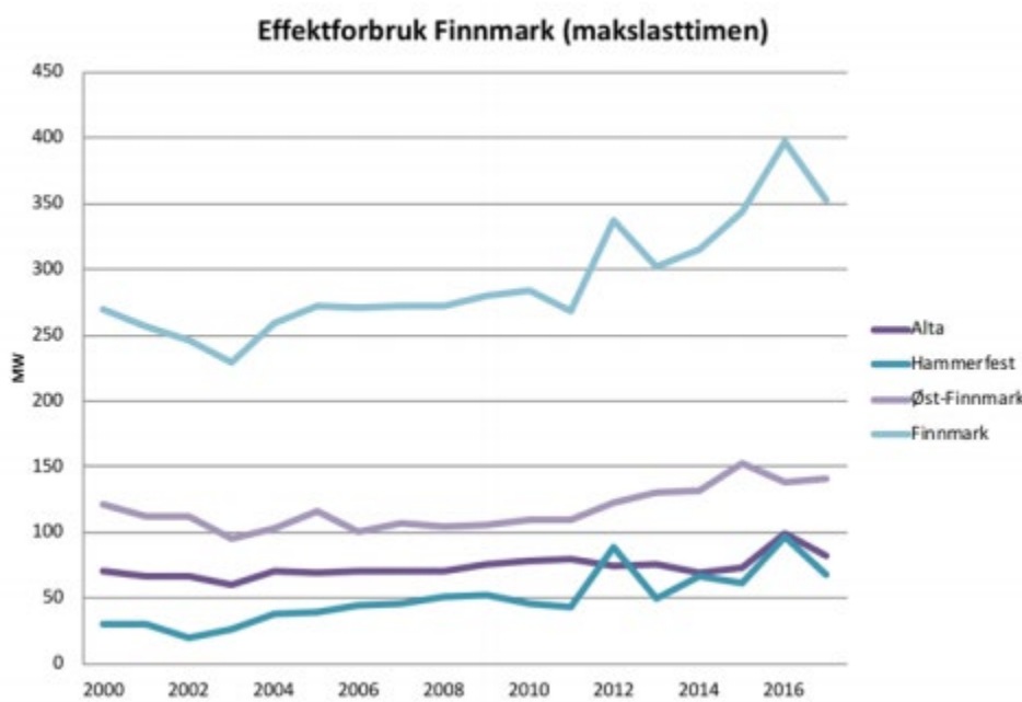
Govus 2-1: Maksimála beaktogolaheapmi Finnmarkkus, ja juohkin golmma oasseguvlui. Gáldu: Statnett (2019).
